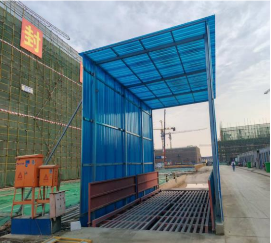
临时洗车池
