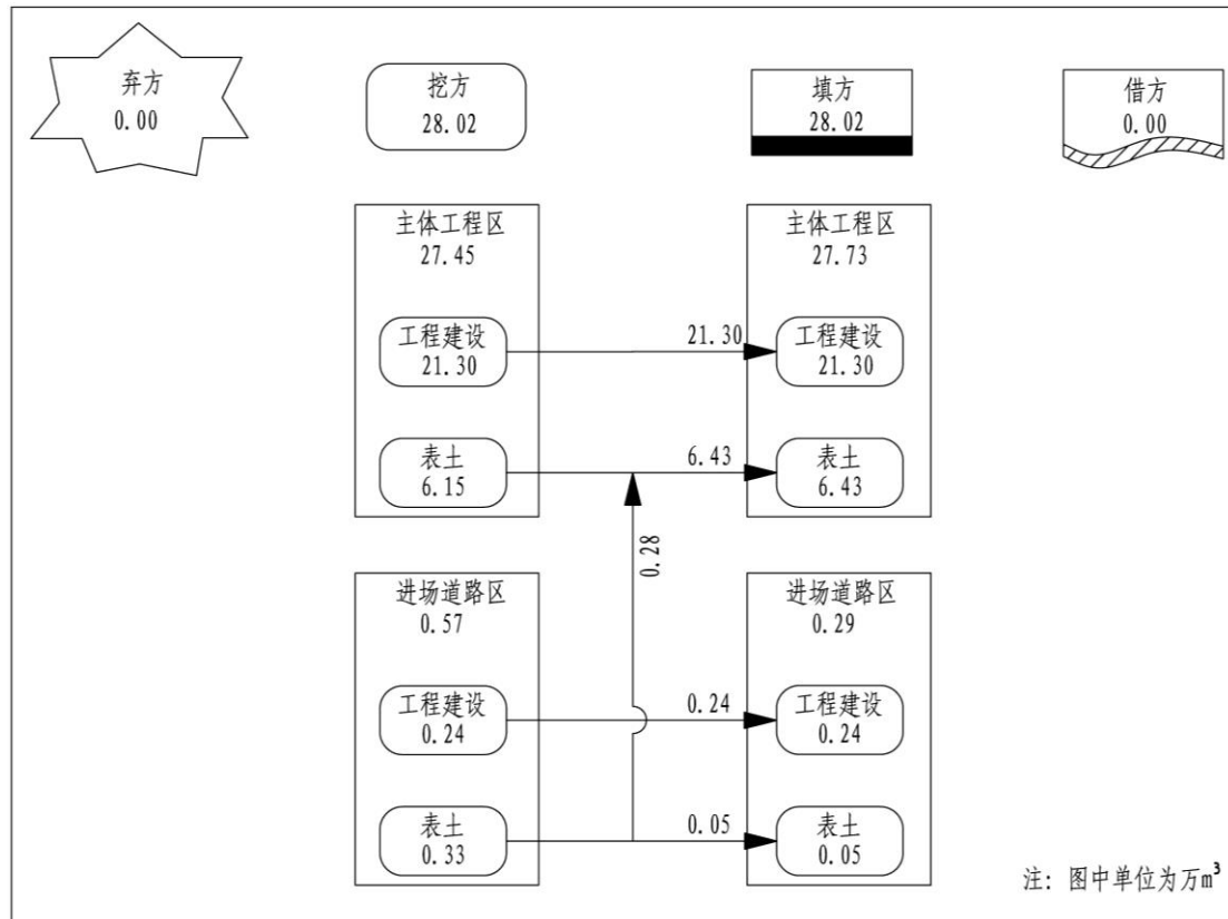
图 2-1 本项目土石方平衡流向框图
